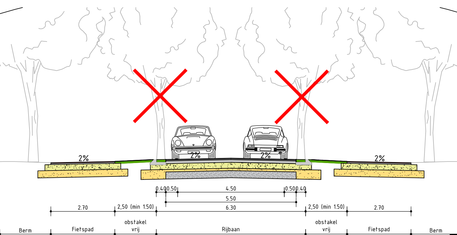
Principeprofiel Heikantstraat Schaal 1 : 100
