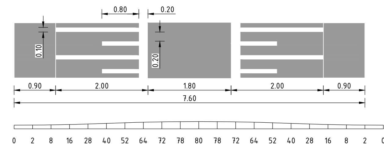
Principe detail drempel 60 km/h 8 cm Schaal 1 : 50
