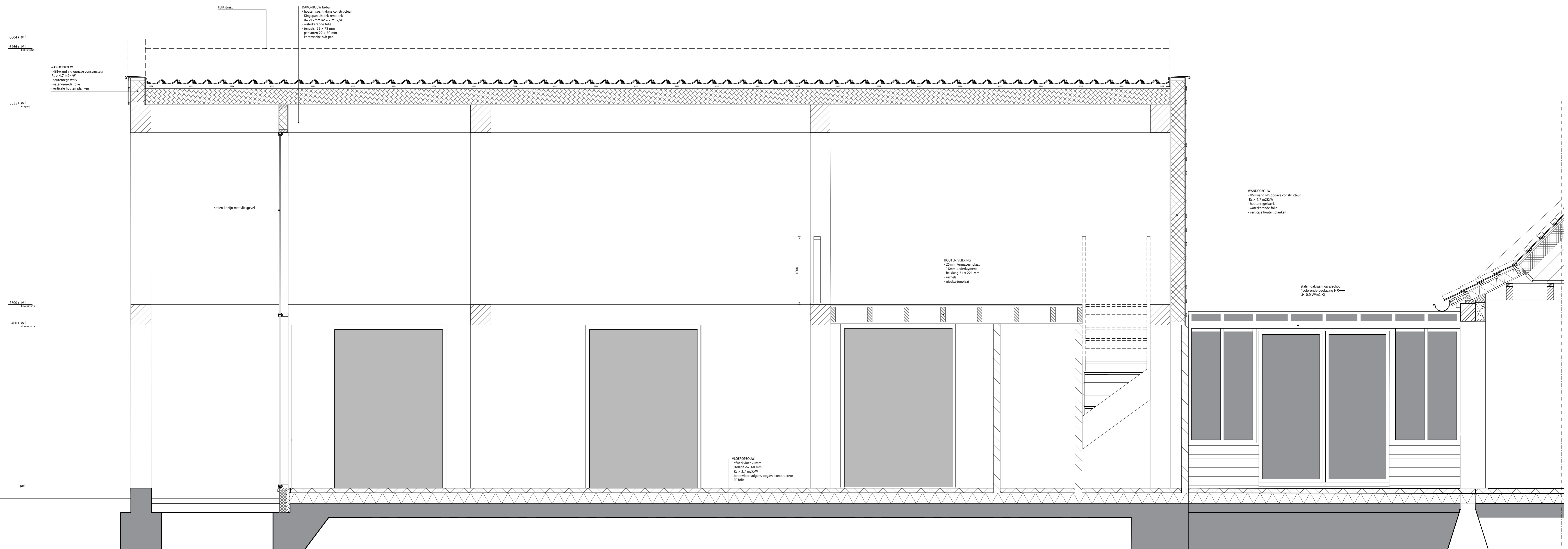
DOORSNEDE D
