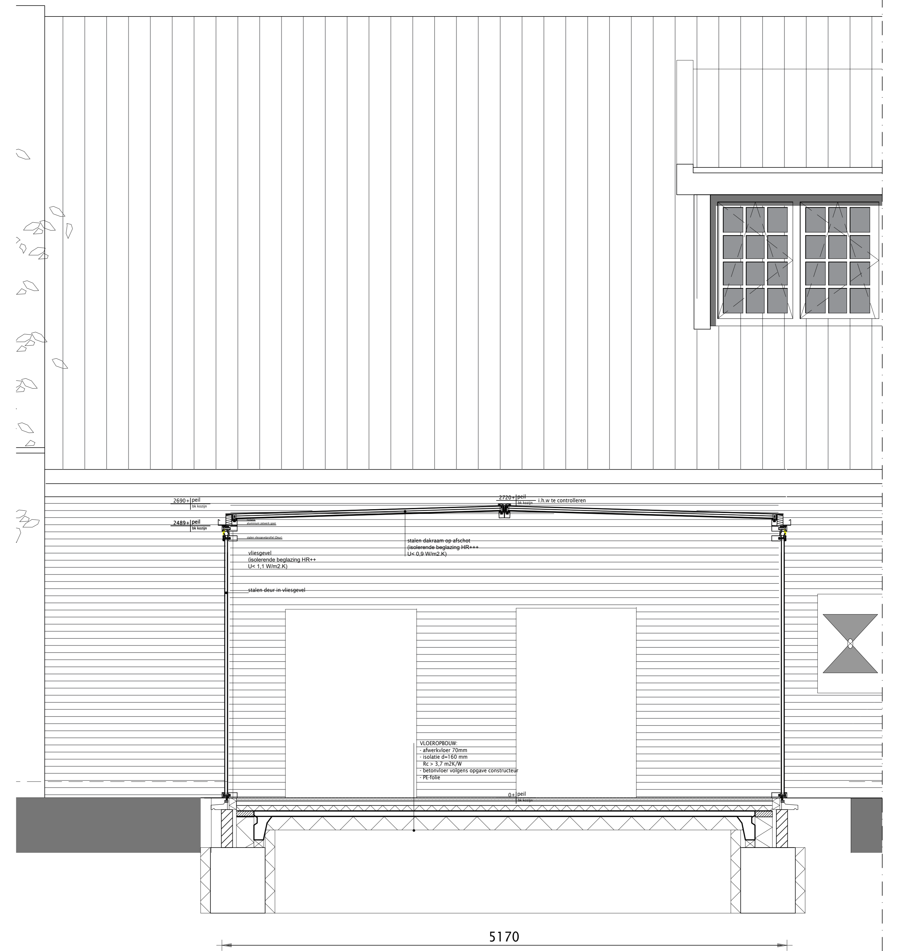
DOORSNEDE C
