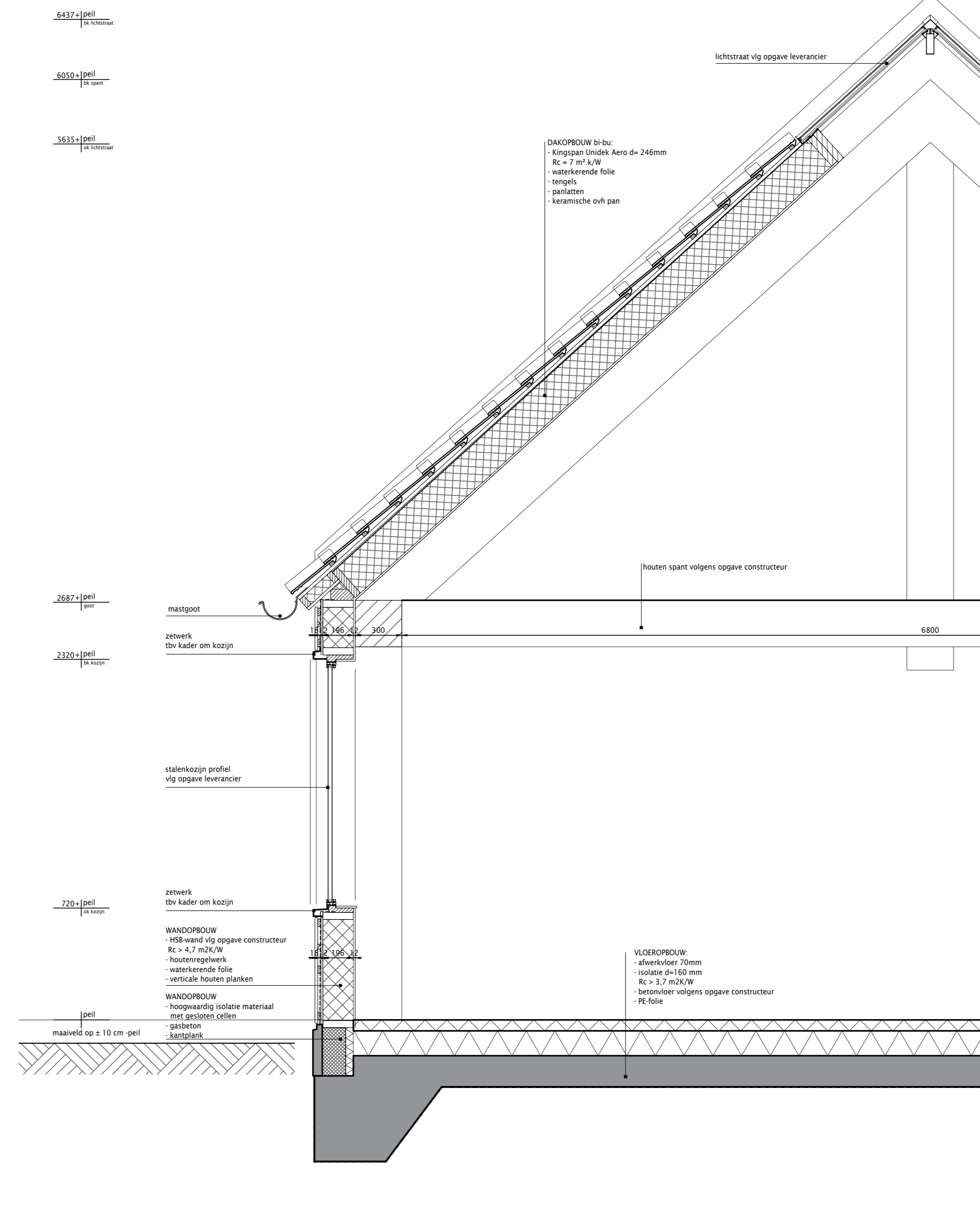
DOORSNEDE B
